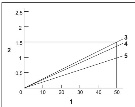
1. Fréquence d'agrafage (fois/min) 2. Sortie d'air du compresseur par minute (CFM (ft³/min)) 3. 0,83 MPa (120 PSIG) 4. 0,66 MPa (95 PSIG) 5. 0,49 MPa (70 PSIG)
